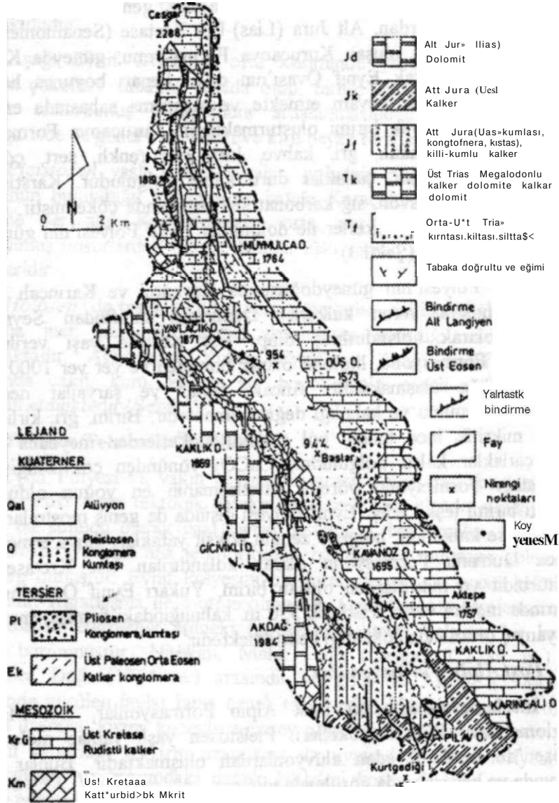
Şekil: 3 EYNİF POLYESİ'NİN JEOLJİ HARİTA5I
